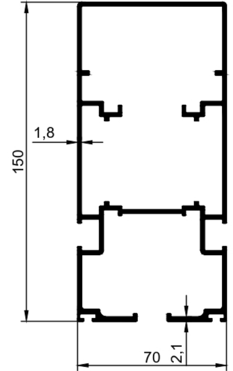
0222 4,338 Kg/m 70'LİK ÇİFT KANAL
