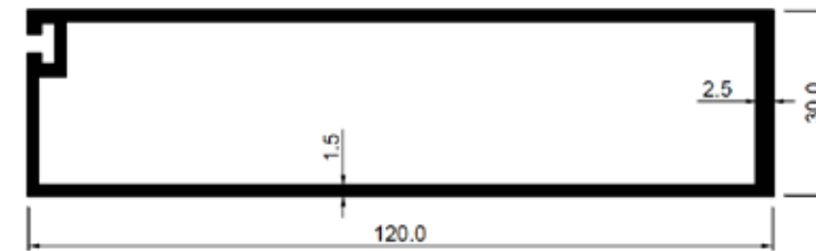
0074 1,315 Kg/m 120X30 TRAPEZ KUTU
