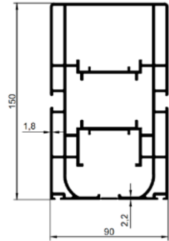
0223 5,430 Kg/m 90'LIK TEK KANALLI
