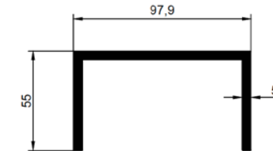
0233 0,917 Kg/m İÇ BAĞLANTI PROFİLİ
