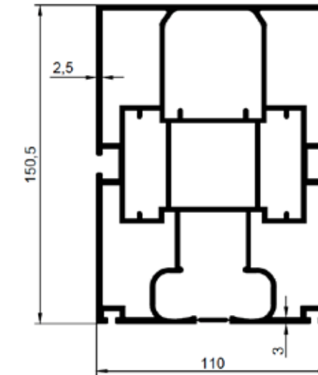
0137 7,142 Kg/m 110'LUK TEK KANALLI
