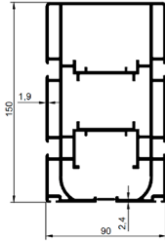
0224 5,543 Kg/m 90'LIK ÇİFT KANALLI
