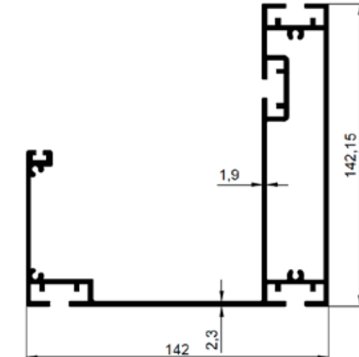
0221 3,807 Kg/m TEKLİ OLUK
