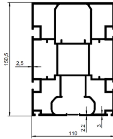
0138 7,091 Kg/m 110'LUK ÇİFT KANALLI
