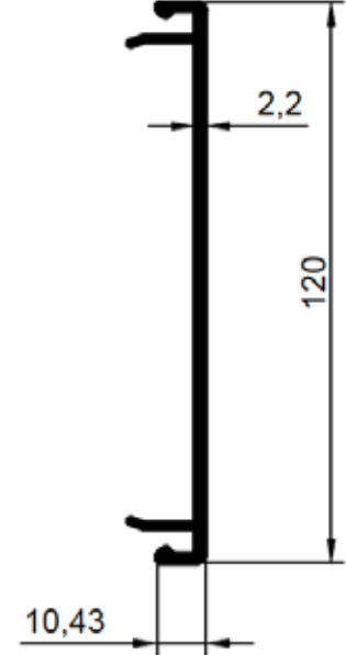
0232 0,917 Kg/m 120X142 KUTU KAPAĞI
