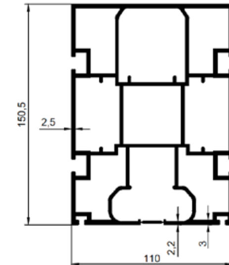
0138 7,091 Kg/m 110'LUK ÇİFT KANALLI
