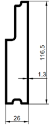
0227 1,366 Kg/m OLUK EKİ
