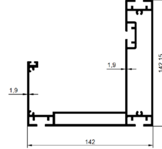
0220 4,100 Kg/m ÇİFTLİ OLUK
