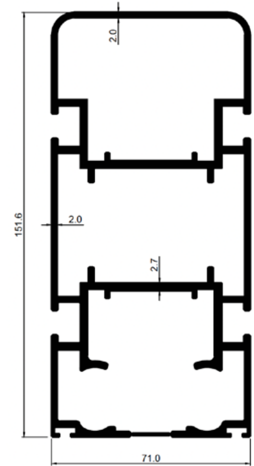
0131 4,283 Kg/m 70'LİK ÇİFT KANALLI RAY
