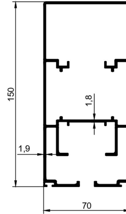
0229 3,170 Kg/m 70'LİK KANALSIZ RAY
