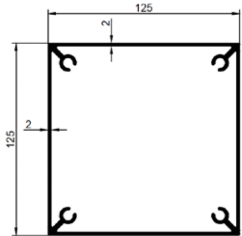
0162 3,666 Kg/m 125x125 DİREK
