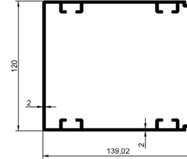
0231 2,715 Kg/m 120X142 KUTU
