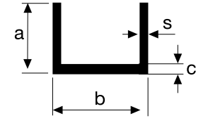
U PROFİLLERİ U Profiles
